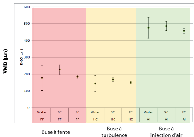
Figure : Effet du type de buses, adjuvant et formulation de phenmediphan - 4.45%w/v (SC or EC) sur la taille des gouttes (moyenne +/- écart type). Source : (Stainier et al, 2006) repris par M. AL HEIDARY, J.P. DOUZALS, C. SINFORT and A. VALLET UMR ITAP, IRSTEA 2013 soumis.
